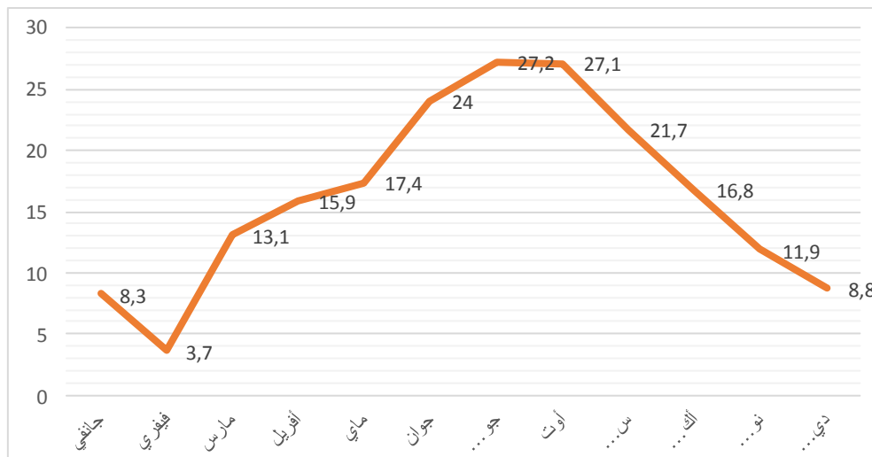
شكل رقم 02: متوسط درجة الحرارة لمدينة تبسة على مدار السنة 2008
