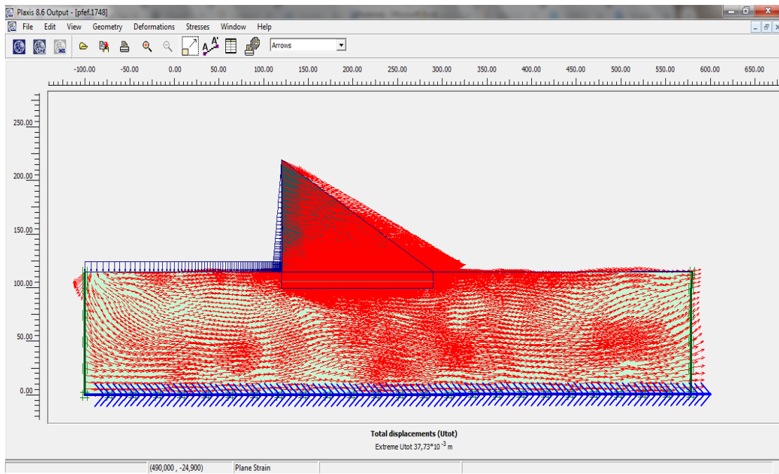
Figure 3.23: Déplacements totaux du barrage
