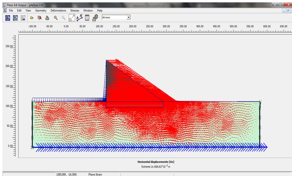
Figure 3.4: Déplacement horizontal
