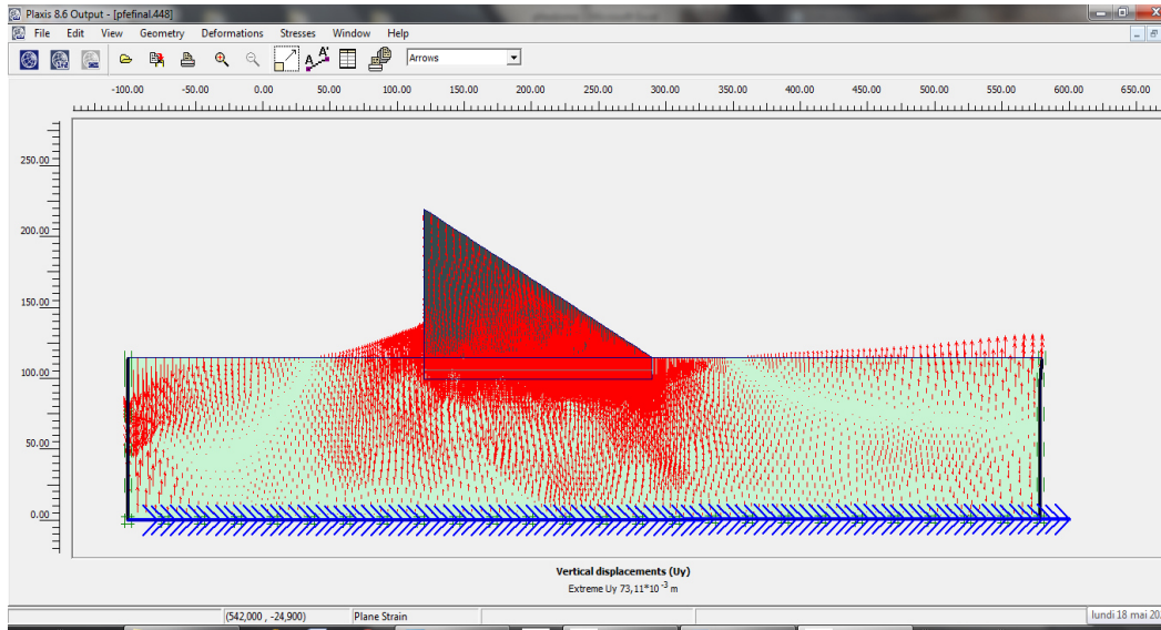
Figure 3.13: Déplacement vertical
