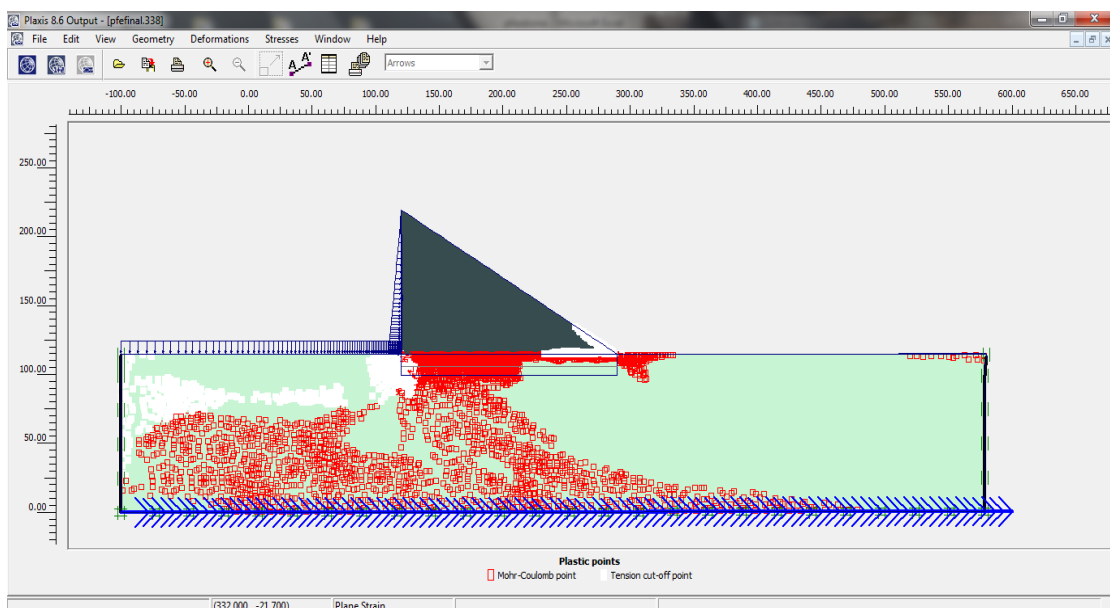
Figure 3.18: Zones plastifiées
