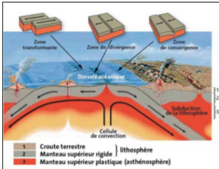
Figure 2.2: Types de frontières de plaques (d’après USGS)
