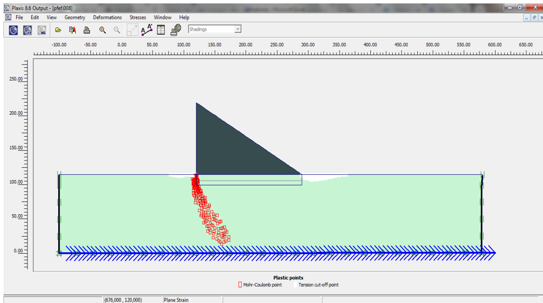
Figure 3.6 : Zones plastifiées
