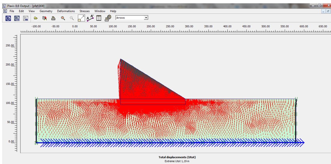
Figure 3.3: Déplacement total
