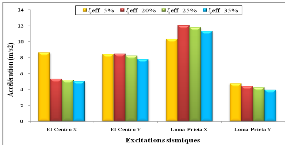
Figure 4.63 : Accélérations du dernier niveau sous différentes excitations sismique et pour différents taux d'amortissement
