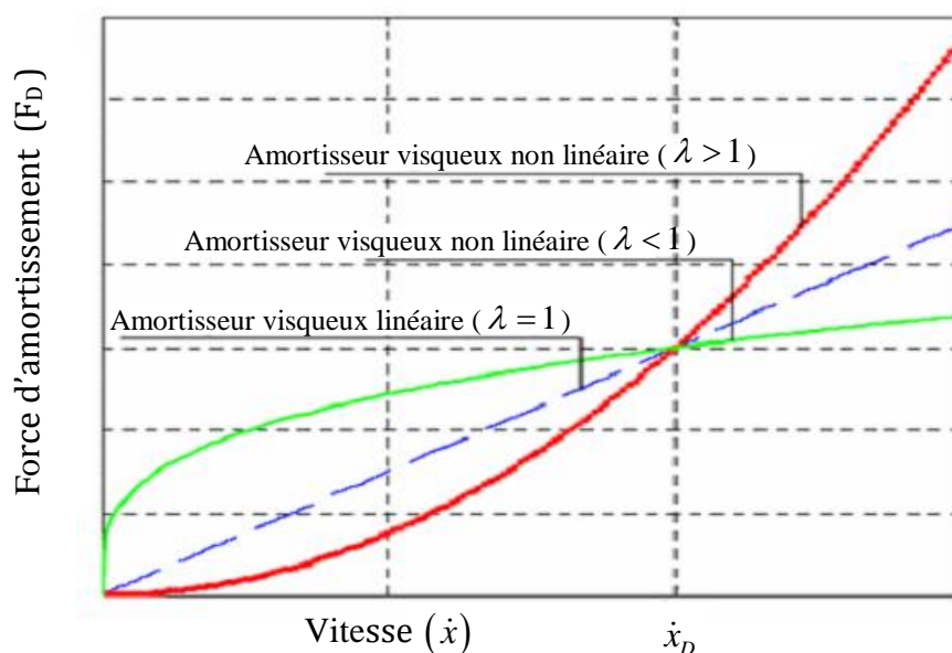
Figure 3.7 : Relation vitesse-force d'amortissement [58]
