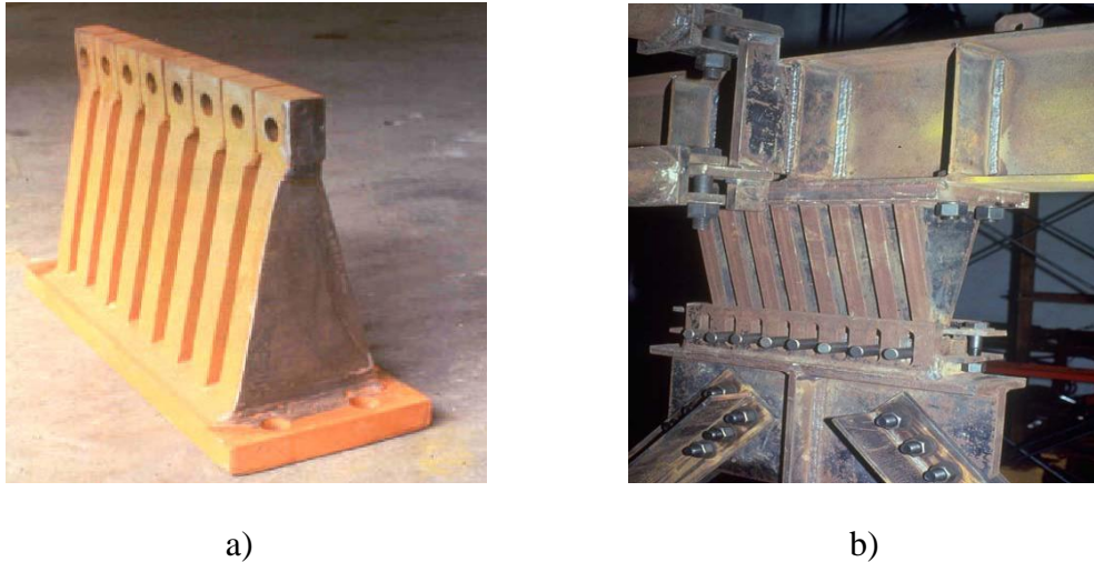
Figure 2.10 : Amortisseur TADAS, a) les plaques triangulaires b) les plaques soudées [19]
