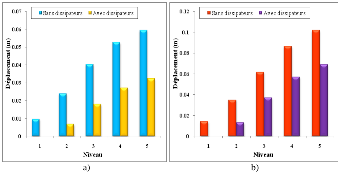
Figure 4.13 : Déplacements des différents niveaux de la structure avec et sans dissipateurs sous le séisme d'El Centro, a) sens X b) sens Y
