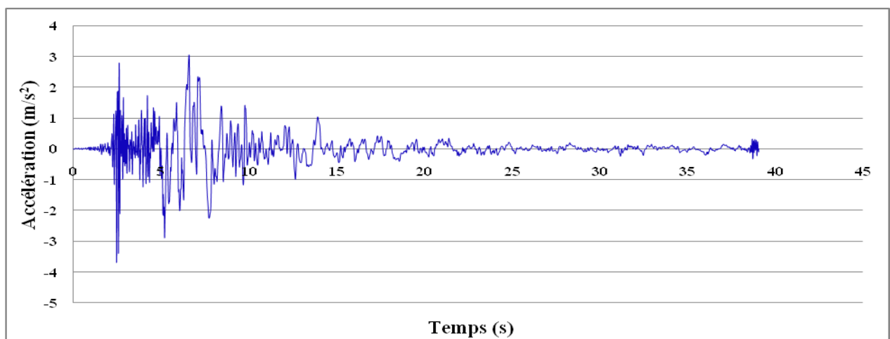
Figure 4.8: Accélérogramme de la composante 140^\circ du séisme d'El Centro avec un PGA= 0.376g
