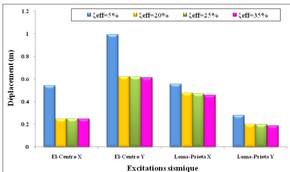
Figure 4.56 : Déplacement du dernier niveau de la structure sous les différentes excitations sismiques et pour différents taux d'amortissement effectif.
