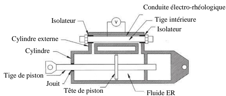
Figure 2.37 : Amortisseur électrorhéologique(ER) [34]
