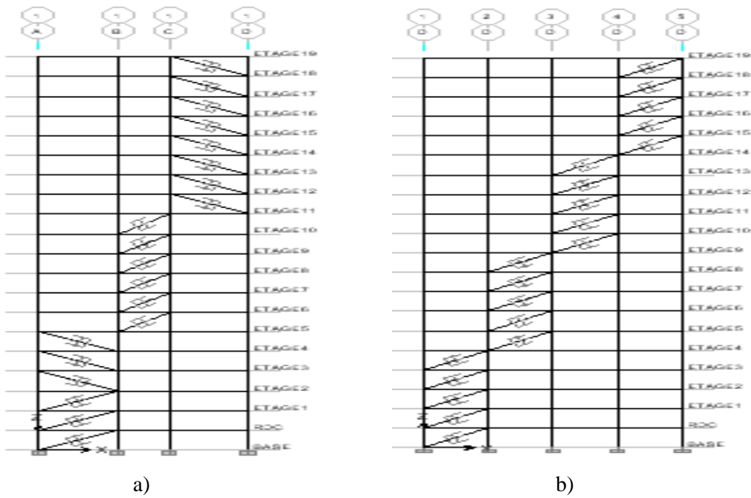
Figure 4.51 : Coupes de La structure avec la nouvelle distribution des dissipateurs : a) Coupes A-A et A'-A', b) Coupe B-B et B'-B'
