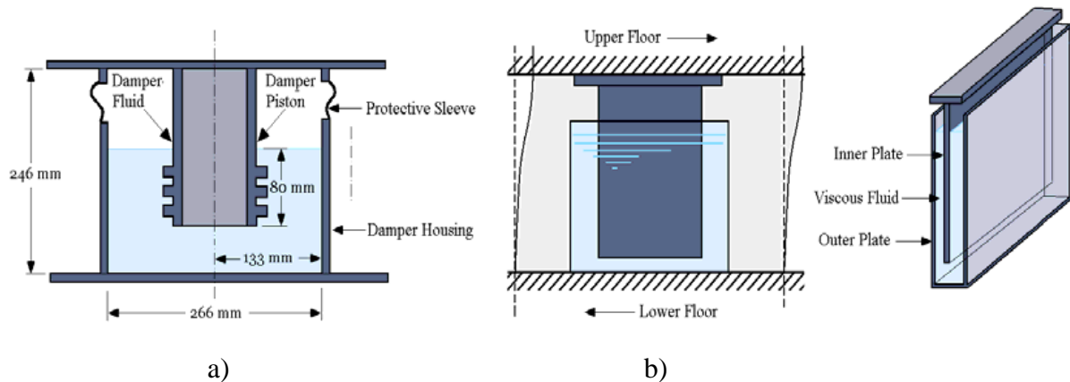
Figure 2.17 : a) ammortisseur à fluide de récipient cylindrique
