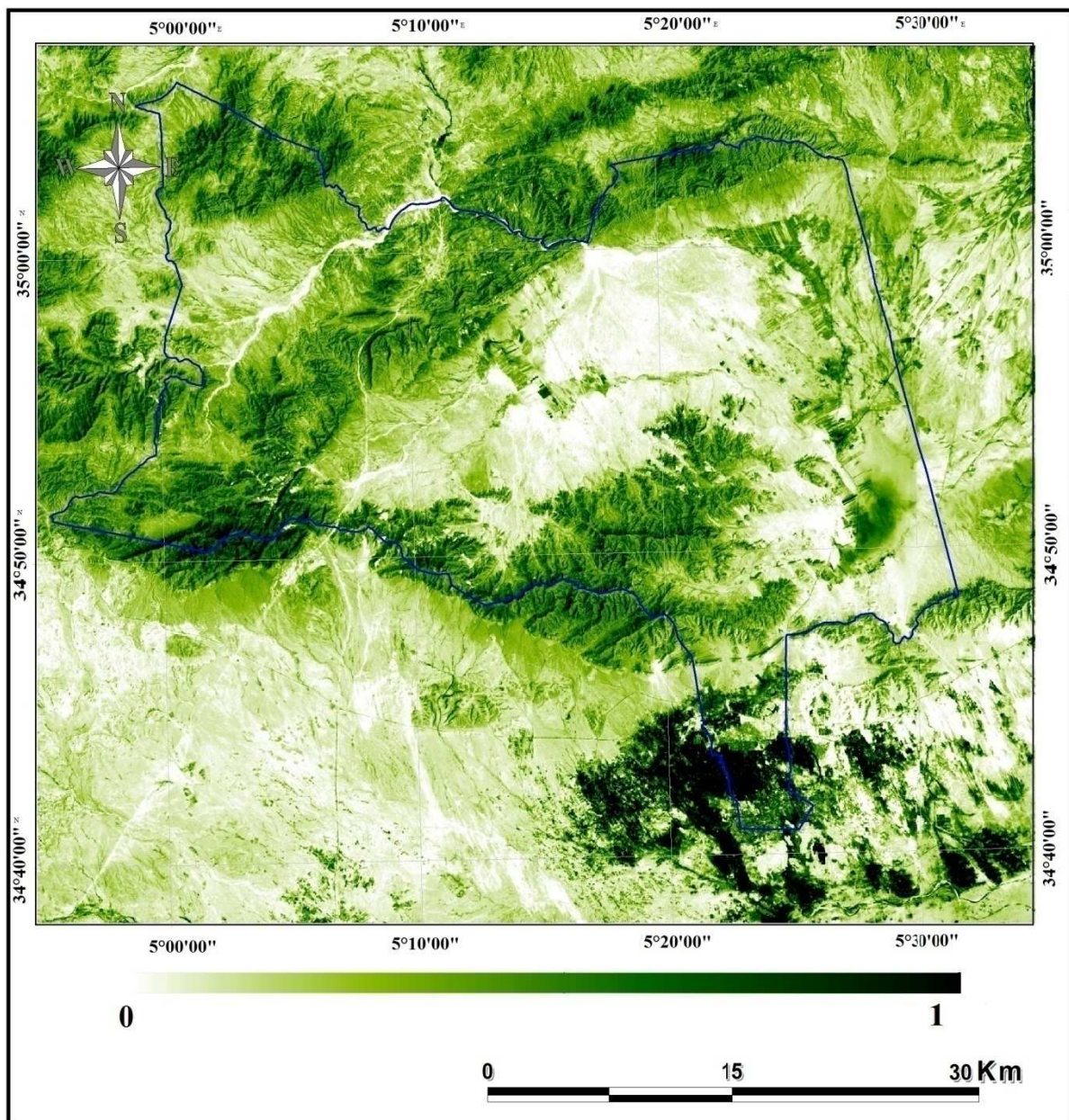
Carte 3 : Carte NDVI de Tolga en 1999.
