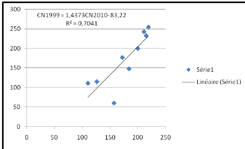
Figure 31: Droite de normalisation du canal TM4
