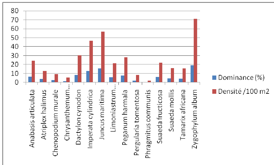
Figure 28 : Dominance et densité pour station 2.
