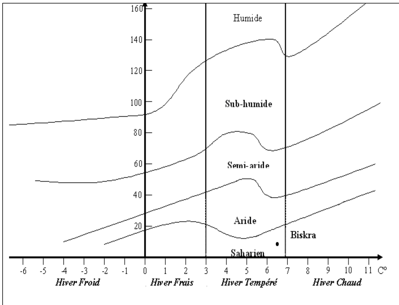
Figure 6: Climagramme d'Emberger de Biskra 1999-2010.
