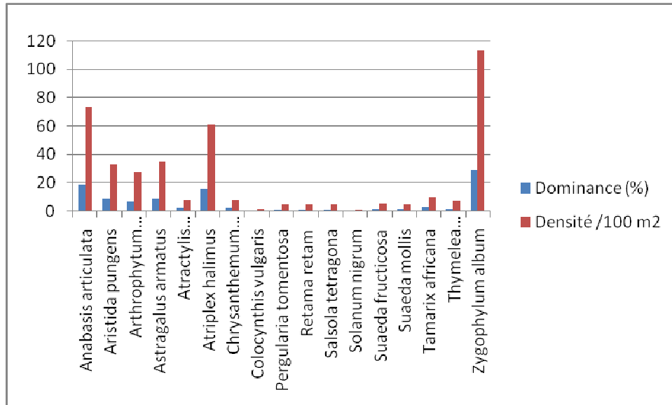
Figure 27 : Dominance et densité pour station1.
