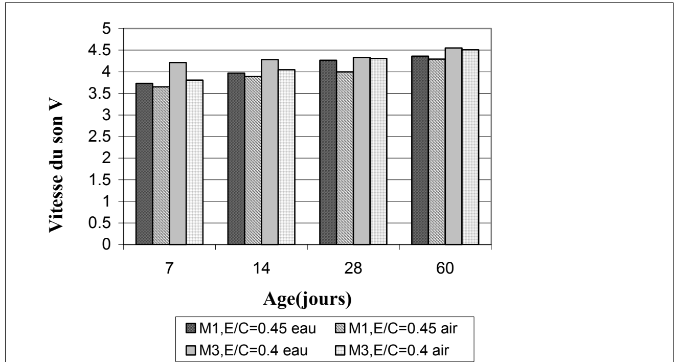
Figure (4.15) : L'influence de type de ciment sur la vitesse du son
