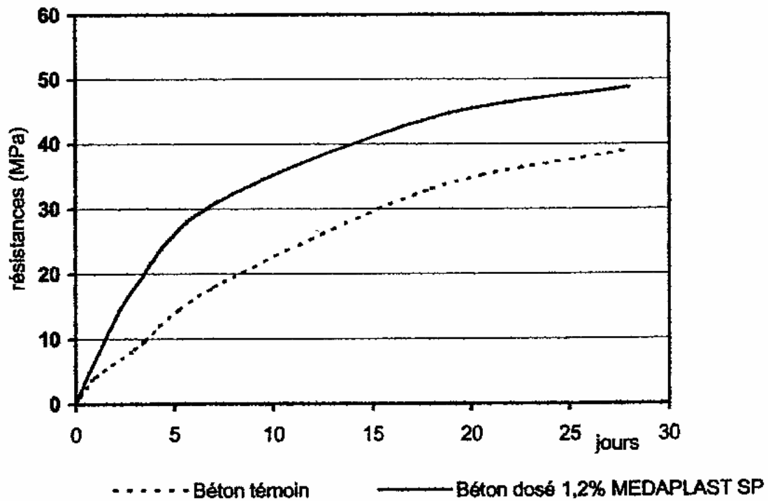
Figure (2.4): Evolution de la résistance à la compression avec le MEDAPLAST (SP) CNERIB(2000)
