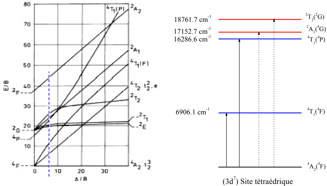
Figure II-23 : Diagramme de Tanabe-Sugano pour l'ion d^7 en symétrie T (ou l'ion d^3 en symétrie octaédrique)
