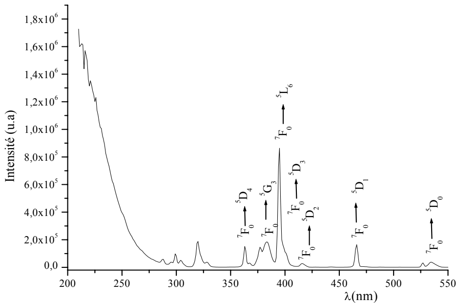
Figure II-36 : Spectre d'excitation à \lambda_{em.} = 612 nm, du cristal \text{NZPO: Eu}^{3+}
