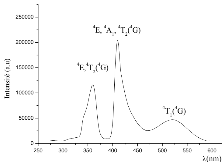
Figure III-7c : Spectres d'excitation enregistrés à T^\circ ambiante pour le verre NZPO dopé de Mn à \lambda_{\text{exc.}} = 409 nm.
