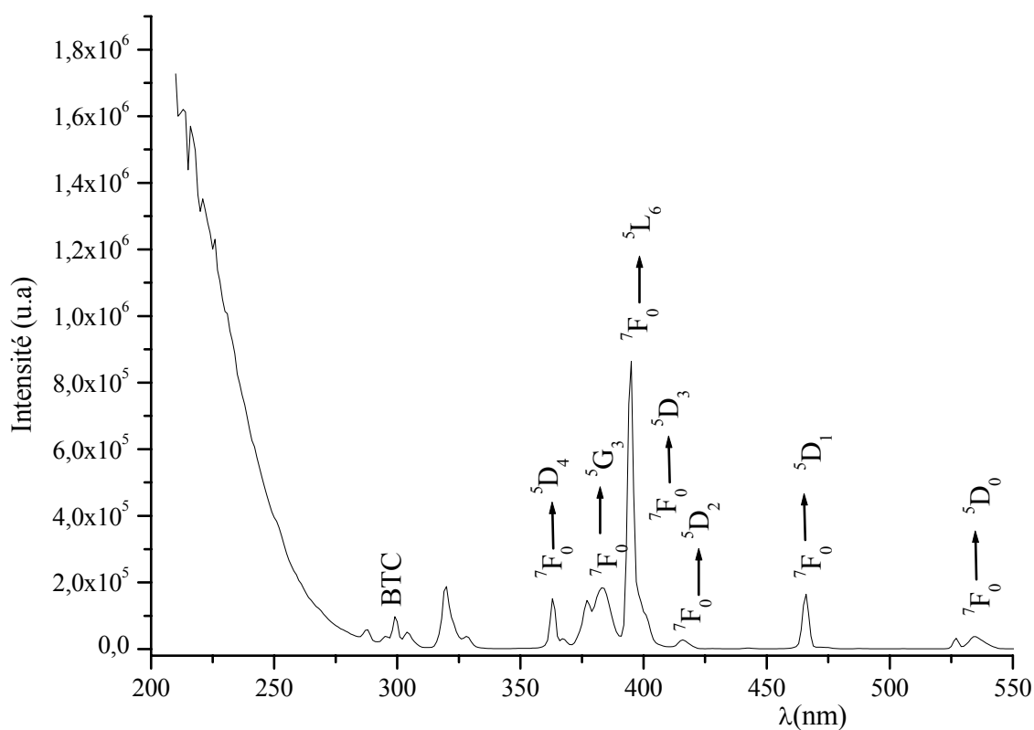
Figure III-9: Spectre d'excitation d'un verre NZPO: \text{Eu}^{3+} 1 mol. % à \lambda_{\text{em.}} = 612 \text{ nm}
