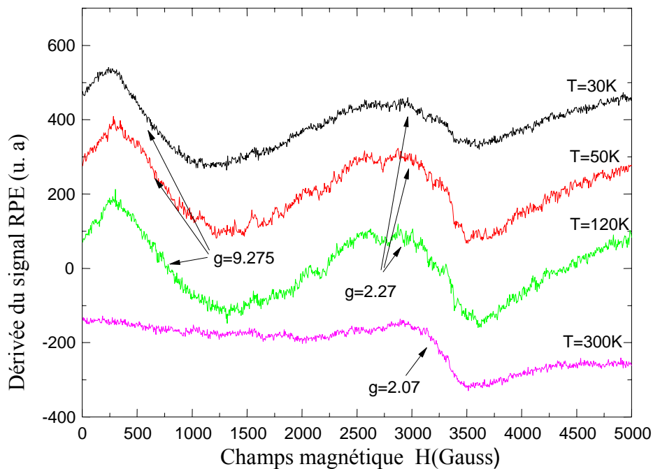
Figure II-20 : Spectres RPE de \text{NZPO: Co}^{2+} mesurés à différentes températures
