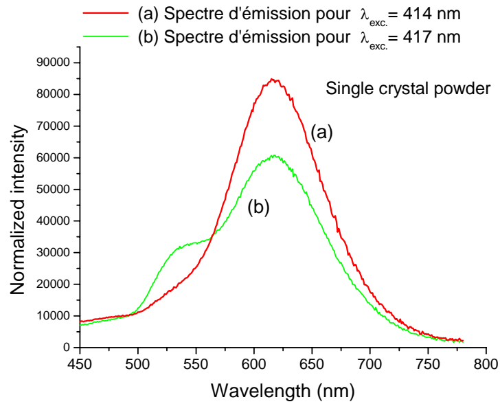
Figure II-30 : Spectres d'émissions enregistrés à température ambiante pour le monocristal \text{NZPO: Mn}^{2+} 0,4 mol. % en poudre:
