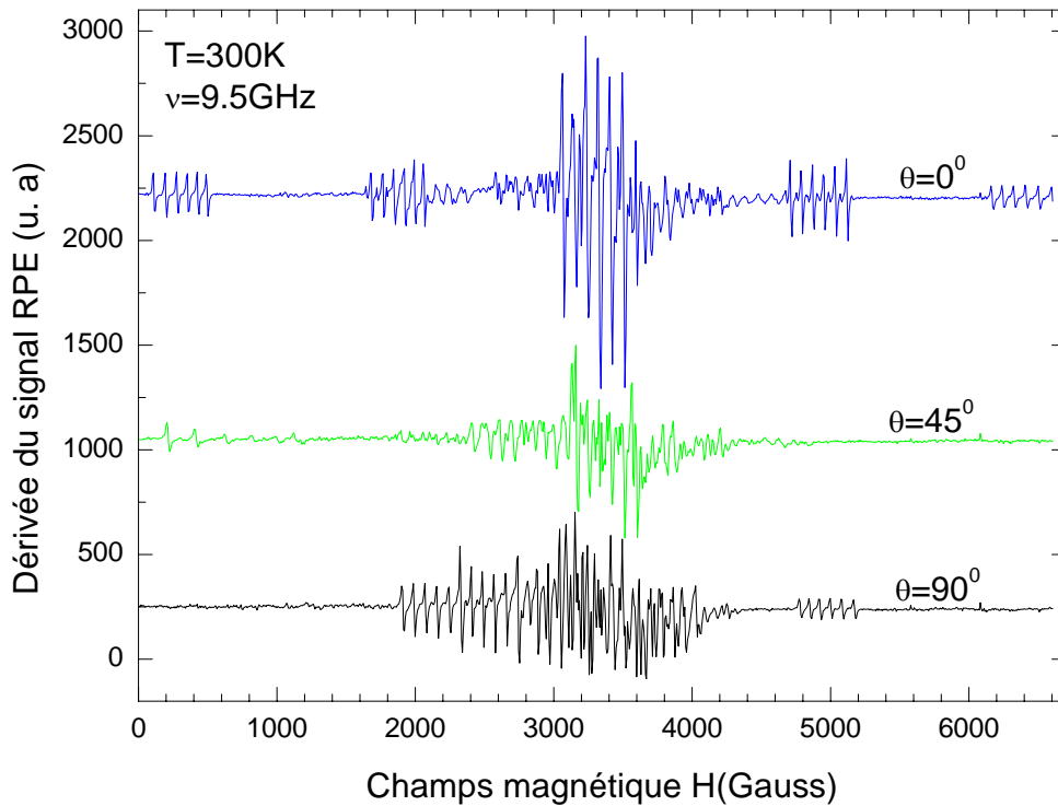
Figure II-13 : Spectres RPE enregistrés à température ambiante dans le plan cristallin xz sur un monocristal de \text{NZPO: Mn}^{2+}
