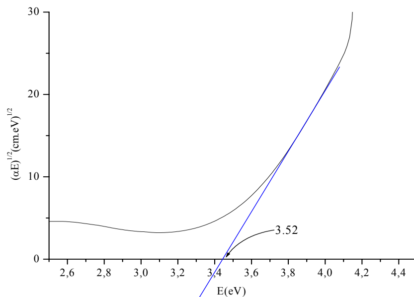
Figure III-12c: Extrapolation de la courbe (\alpha E)^{1/2}(E) de NZPO: \text{Mn}^{2+} dopé 1 mol.%
