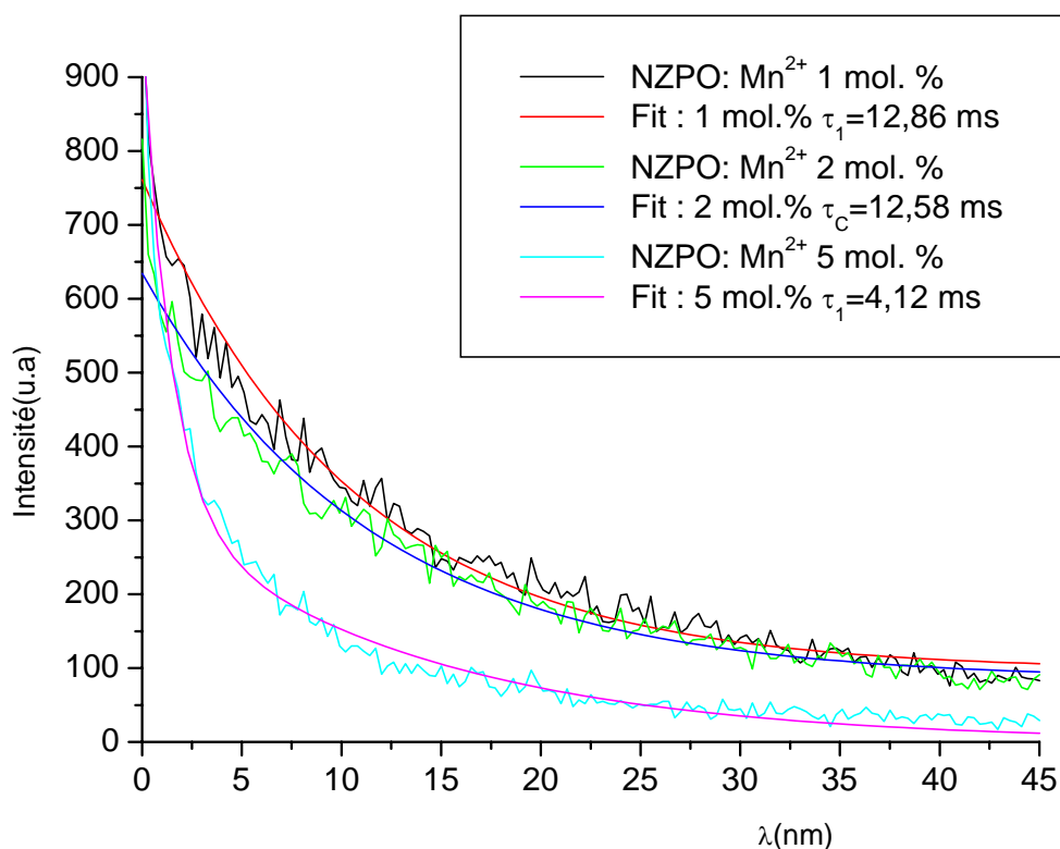
Figure III-13 : Meilleurs ajustements / Spectres du déclin pour verres ( \lambda_{em}=628 nm):
