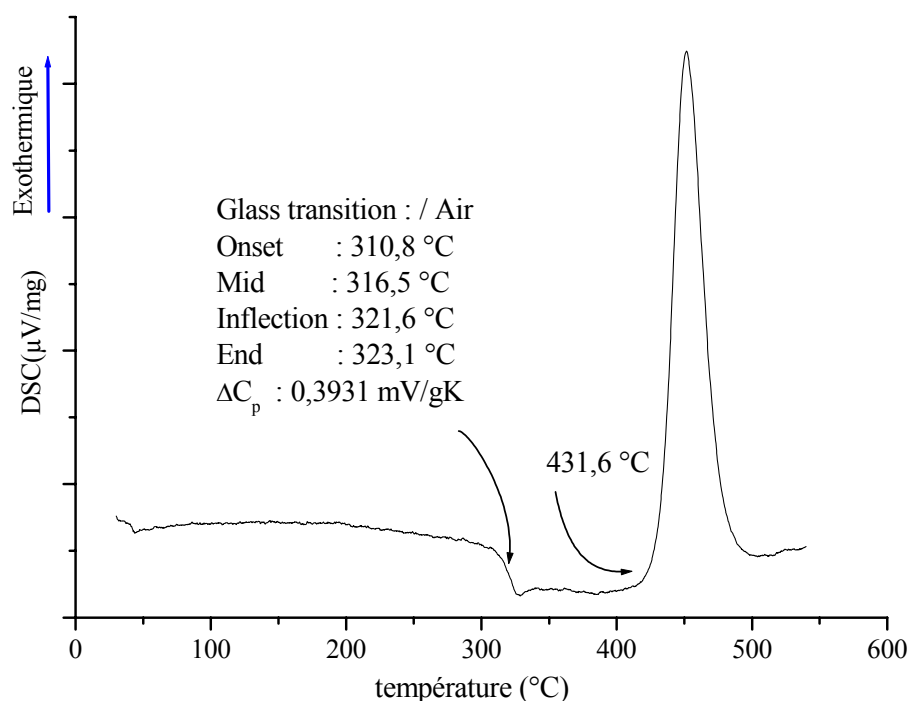
Figure III-2a : ATD d'un verre NZPO: \text{Co}^{2+} 1 mol.%
