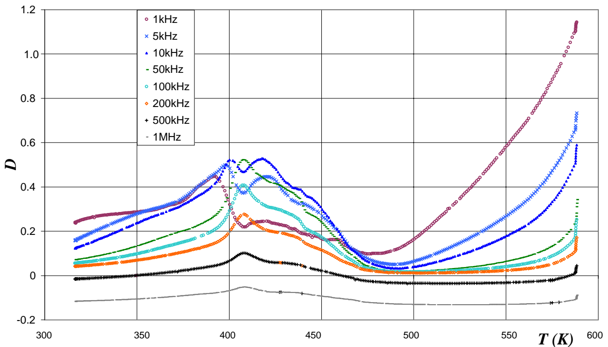
Figure IV-13 : Evolution thermique du facteur de pertes diélectriques D pour un cristal de BTNN16/84 au refroidissement et à diverses fréquences.
