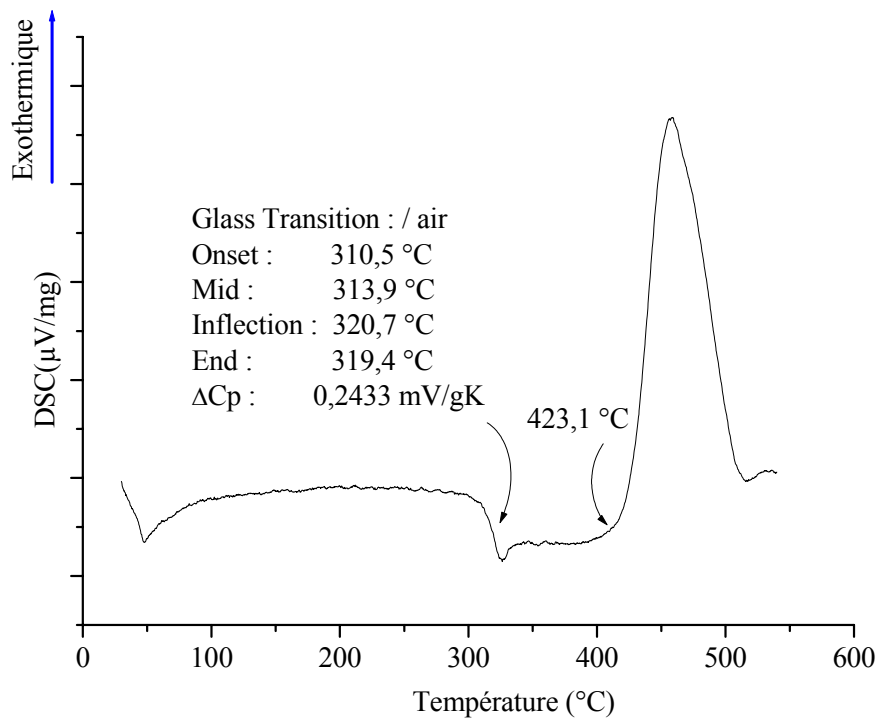
Figure III-2c : ATD d'un verre NZPO: \text{Mn}^{+2} – 1 mol.%
