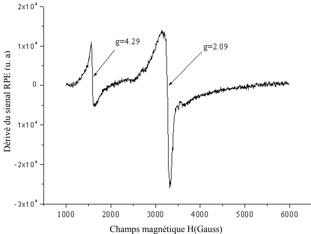
Figure II-21 : Spectres RPE pour le monocristal NZPO: \text{Eu}^{3+} , enregistré à 4 K.
