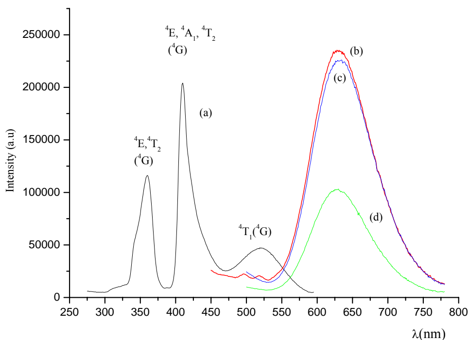
Figure III-8 : Spectres d'émission et d'excitation enregistrés à T° ambiante pour les verres :
