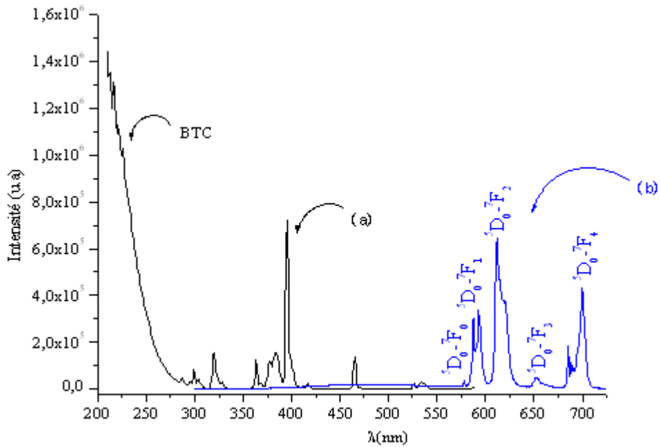
Figure II-35 : Spectres (a) d'excitation à \lambda_{em.} = 612 nm, et (b) d'émission \lambda_{exc.} = 395 nm du cristal \text{NZPO: Eu}^{3+} , à l'air
