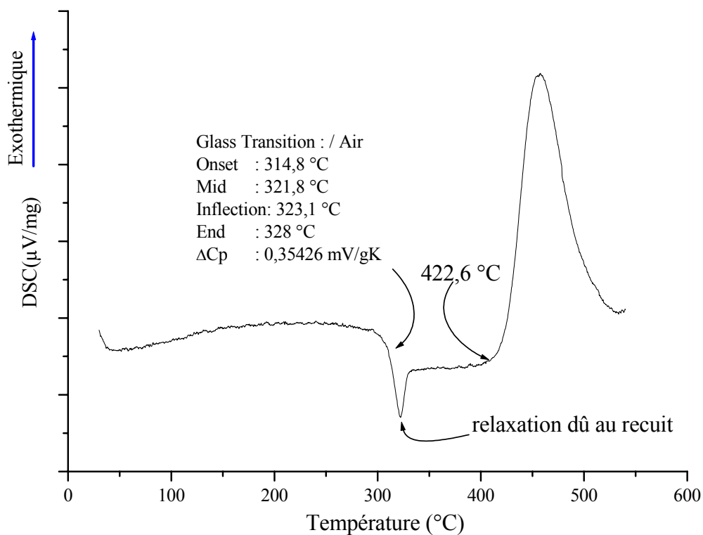
Figure III-2b : ATD d'un verre NZPO: \text{Ni}^{+2} 1 mol.%
