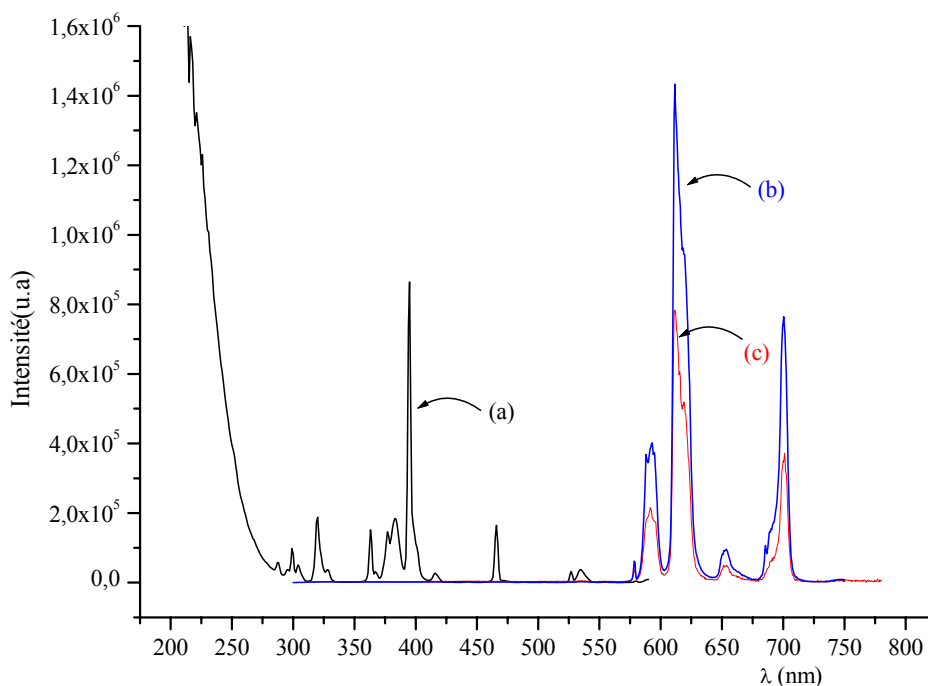
Figure III-11 : Spectres d'émission et d'excitation enregistrés à T^\circ ambiante pour les verres : (a) NZPO: \text{Eu}^{3+} / \lambda_{\text{exc.}}=255 nm ; (b) NZPO: \text{Eu}^{3+} 1 mol.% ; (c) NZPO: \text{Eu}^{3+} 2 % / \lambda_{\text{em}} = 612 nm.
