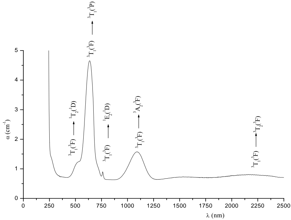
Figure II-24: Spectre d'absorption du cristal NZPO: \text{Ni}^{2+} épaisseur 0,129cm, à température ambiante.
