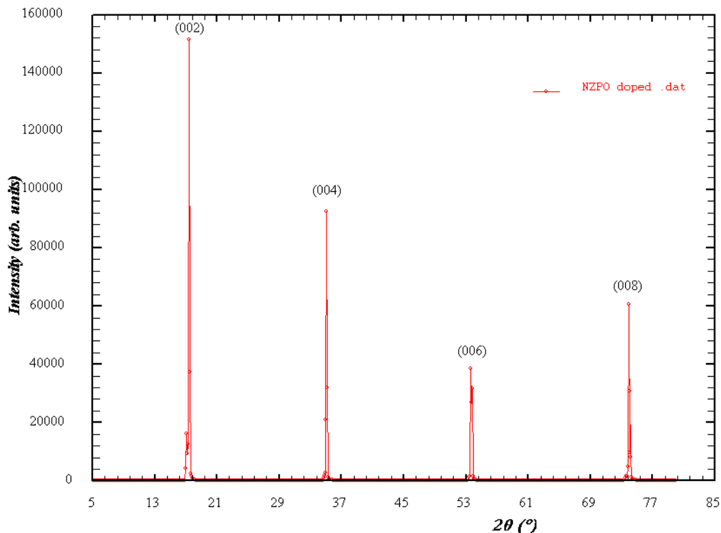
Figure II-10 : Diagramme de diffraction X d'une plaquette découpée dans le monocristal NZPO : dopé \text{Co}^{2+} selon c.
