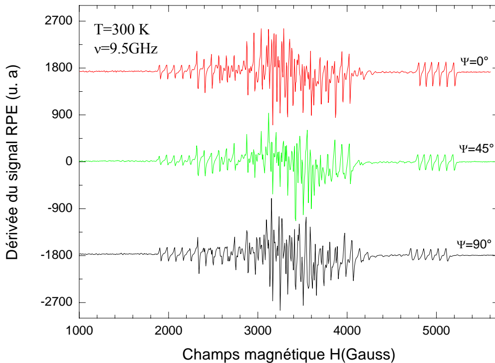
Figure II-14 : Spectres RPE enregistrés à température ambiante dans le plan cristallin xy sur un monocristal de \text{NZPO: Mn}^{2+}
