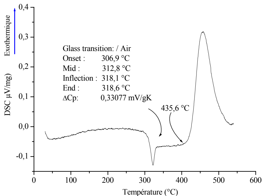
Figure III-2d : ATD d'un verre NZPO: \text{Eu}^{+3} – 1 mol.%
