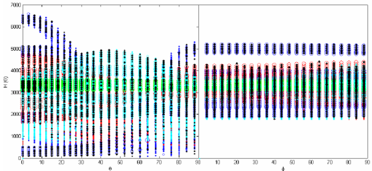
Figure II-17 : Dépendance angulaires théorique dans les plans zx et xy pour NZPO : \text{Mn}^{2+} (Les points tracent les résultats expérimentaux).
