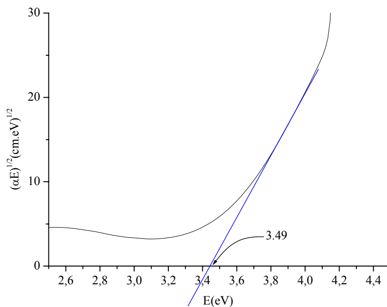
Figure III-12d: Extrapolation de la courbe (\alpha E)^{1/2}(E) de NZPO: \text{Eu}^{3+} dopé 1 mol.%
