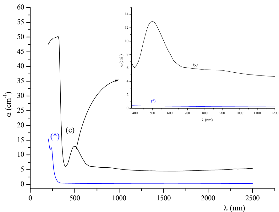
Figure III-6c: Spectres d'absorption des verres:
