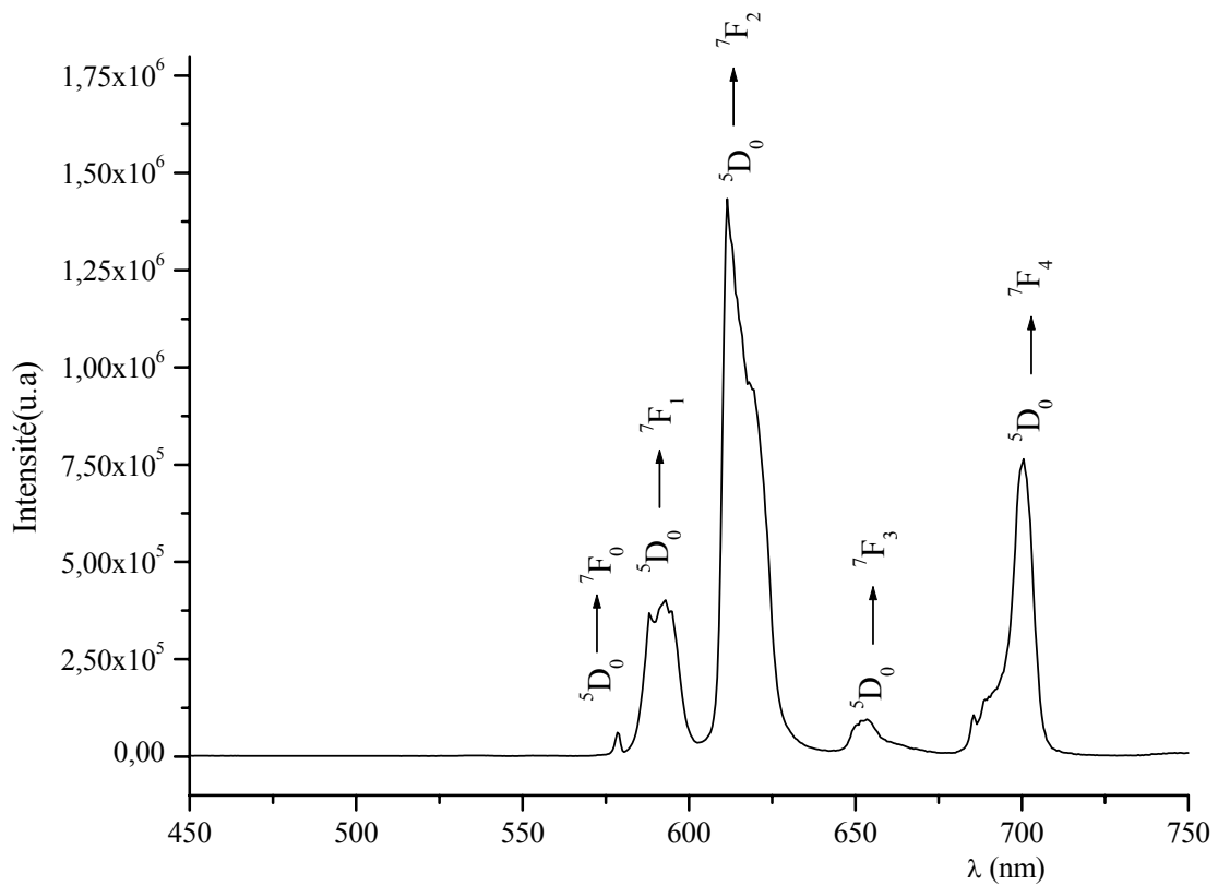
Figure III-10: Spectre d'émission d'un verre enregistré à T^\circ ambiante de NZPO: \text{Eu}^{3+} 1 mol. % à \lambda_{\text{exc.}}=255\text{nm}
